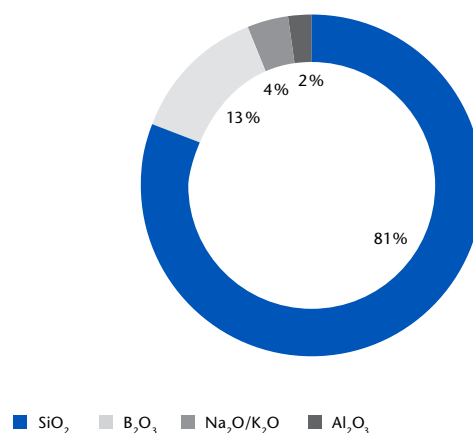
TEMPAX Float®の化学組成
